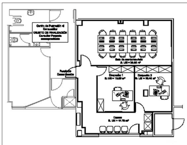
Uno de los planos del proyecto de adaptación de las nuevas dependencias de Consumo
